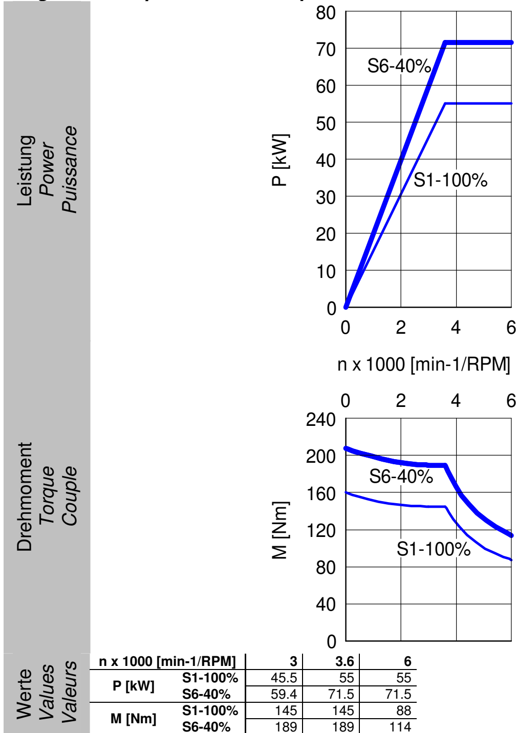
Leistungs- und Drehmomentdiagramm Power- and Torque-Diagram Diagramme de puissance et couple
